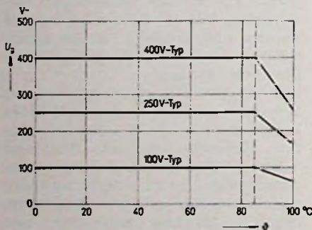
Bild 1.50. Dauergrenzspannung U_g bei Betrieb mit Gleichspannung in Abhängigkeit von der Temperatur (Siemens)
